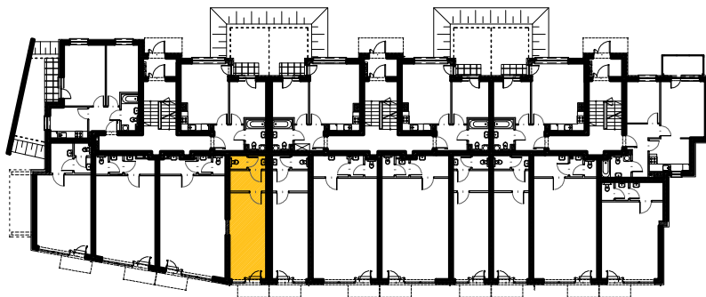
RZUT PARTERU
